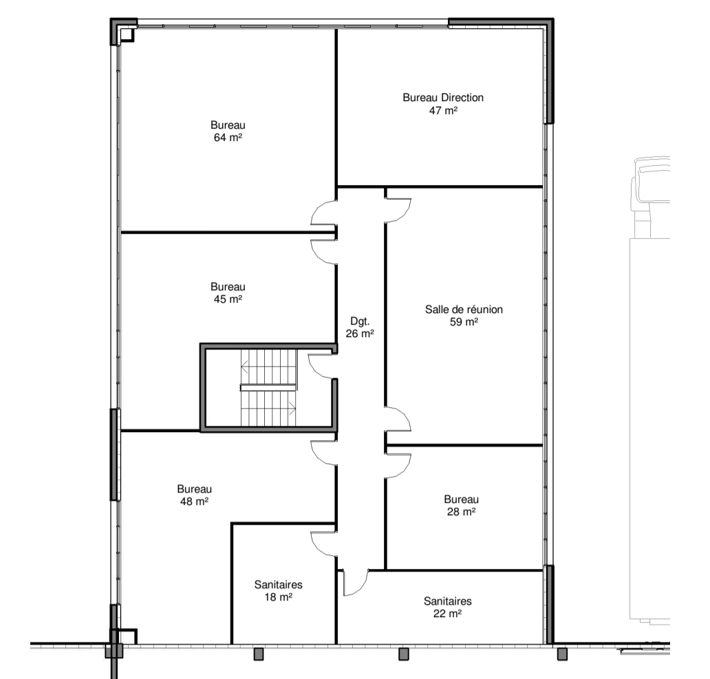
01 - Etage 1 - 1-200 Ech : 1:200
